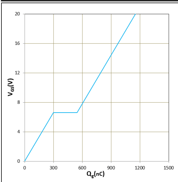
Figure 12. V_{GS} vs Q_g T_j = 25^\circ\text{C} , I_D = 375\text{A} , V_{DS} = 920\text{V}
