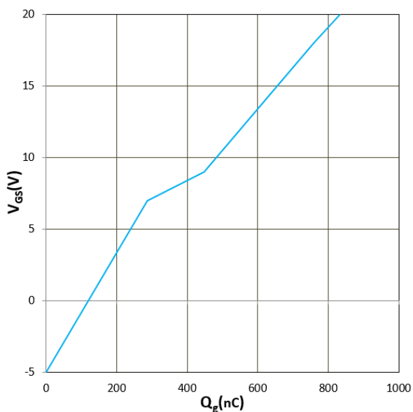
Figure 14. V_{GS} vs Q_g T_J = 25^\circ C , I_{GS} = 4mA
