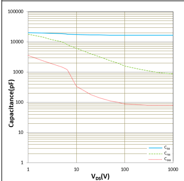
Figure 22. C_{iss} , C_{oss} , C_{rss} vs V_{DS} T_j = 25^\circ C
